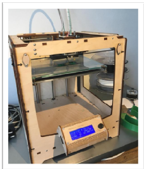
Imprimante 3D munie d'une bobine avec des fils en fibre végétaux
